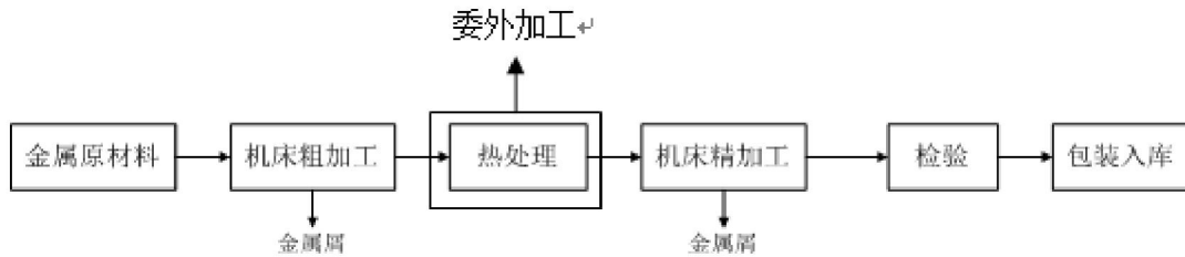
图 2-1 生产工艺流程图
